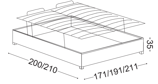
BASE CON RETE SOLLEVABILE A DUE MOVIMENTI SMONTABILE
